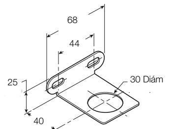
Escuadra (para el regulador y cuerpo del filtro/lubricador) P31KA00MR
